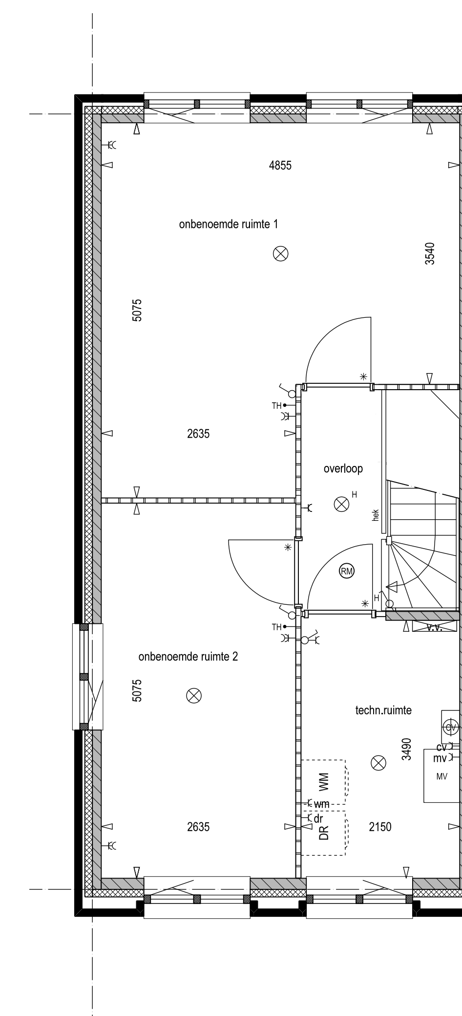
4e verdieping type O getekend type Oa - optie inrichting 4e verdieping
