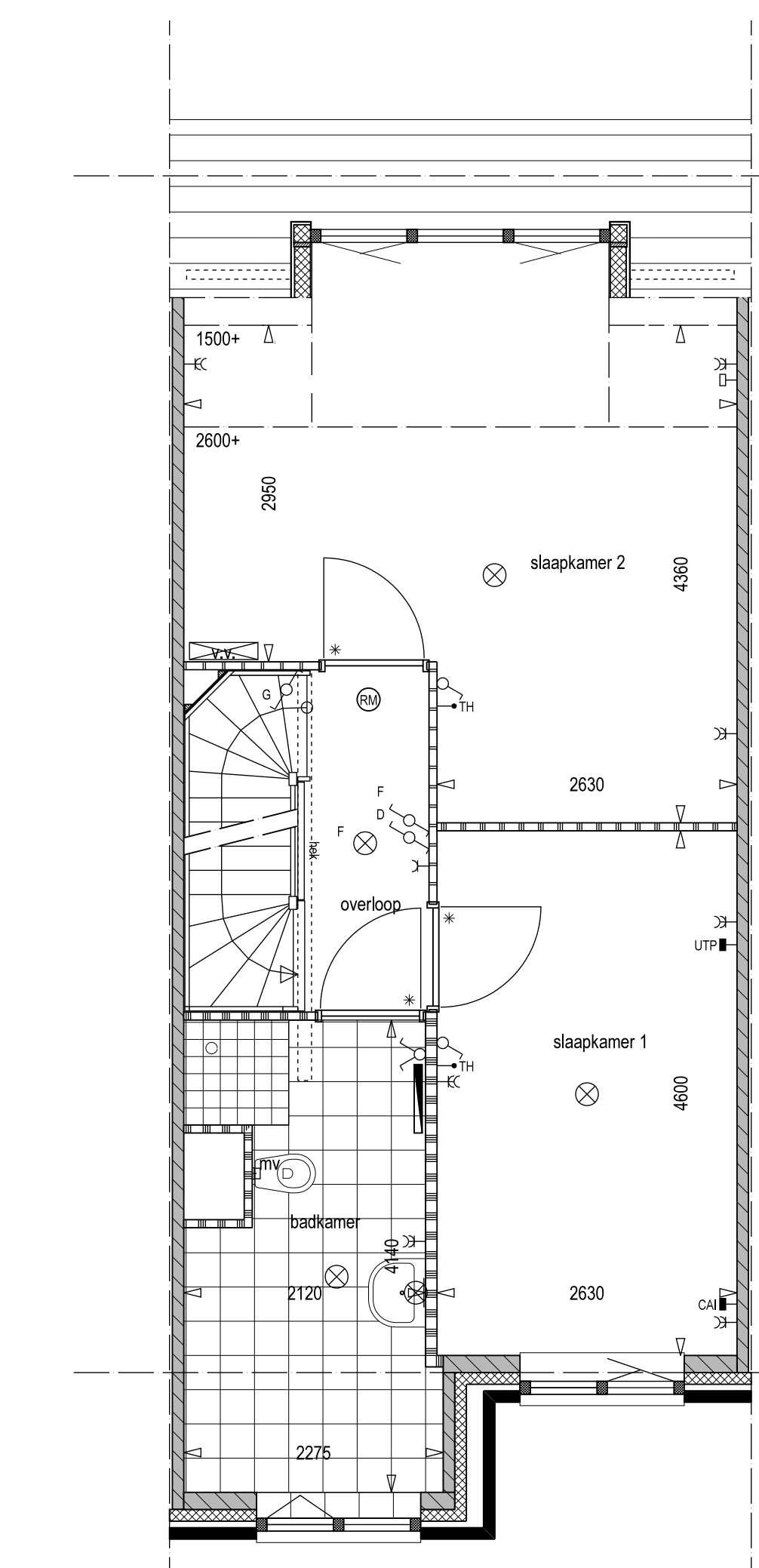
2e verdieping type L, M en N getekend type L1 - optie dakkapel achtergevel 2e verdieping
