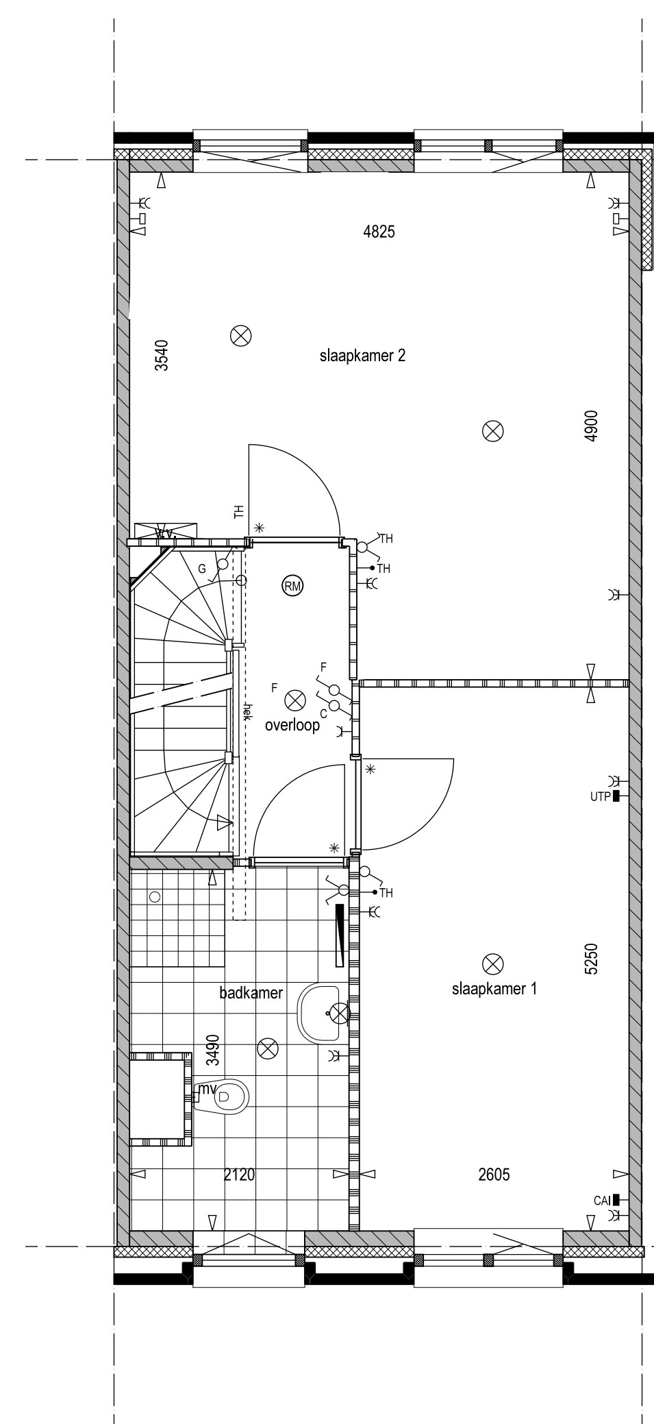
2e verdieping type K en O getekend type K1 - optie 2 slaapkamers (pv 3)
