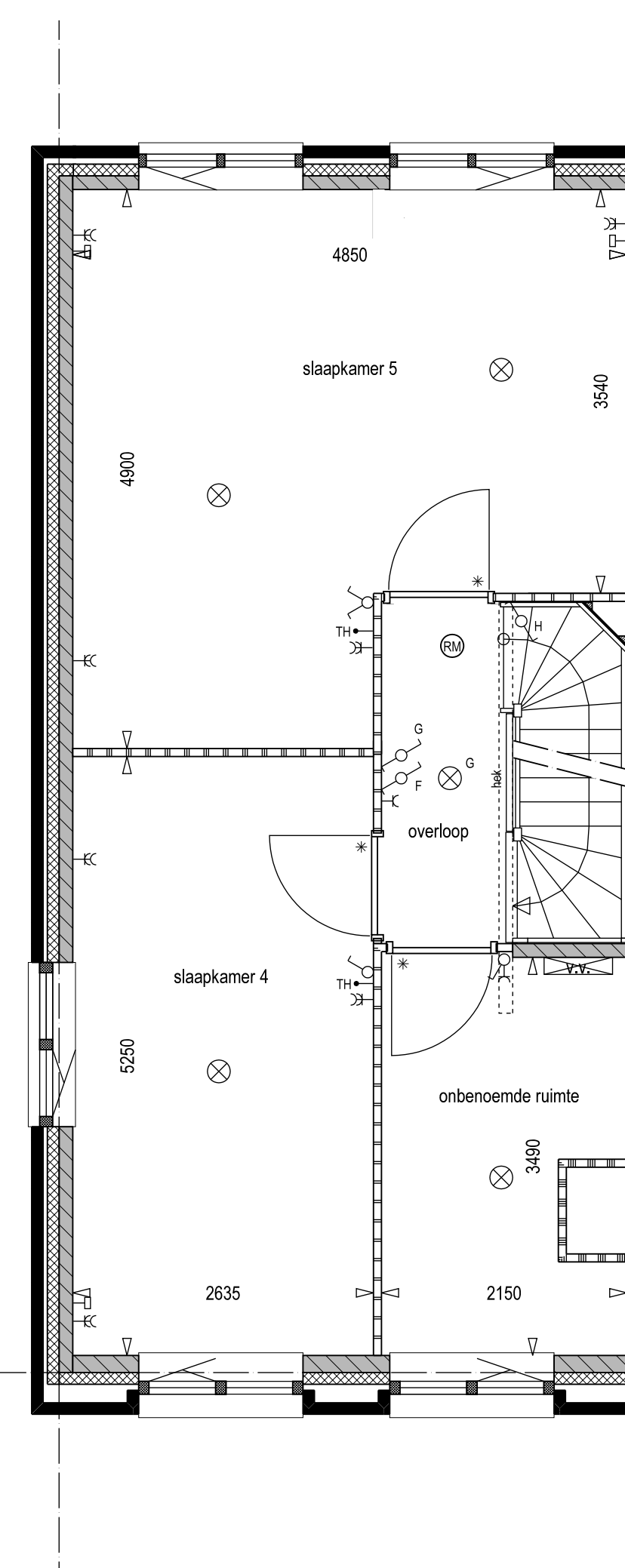
3e verdieping type O getekend type Oa - optie 2 slaapkamers (pv 3)
