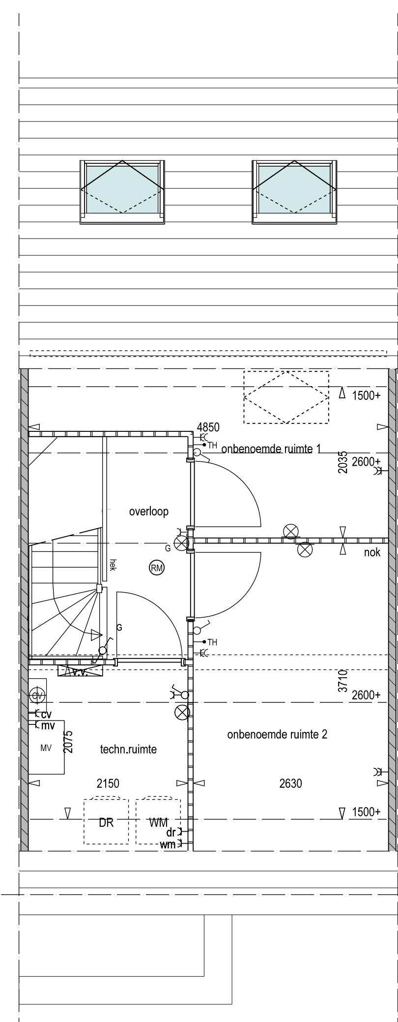
zolder type L, M en N getekend type L1 - optie indeling zolderverdieping
